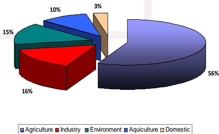
Utilización agua por sectores 2010
