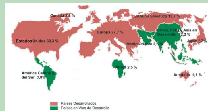
Fig. 2.2.- Contribución al calentamiento global del planeta expresado en porcentaje. Nota: Las áreas son proporcionales a las emisiones históricas de CO 2 de 1990 a 1999 provenientes de la utilización de combustibles fósiles. Fuente: World Resources Institute , 2002. Elaboración propia a partir del mapa Contributions to Global Warming .
